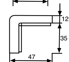
Eckschutz Typ H
