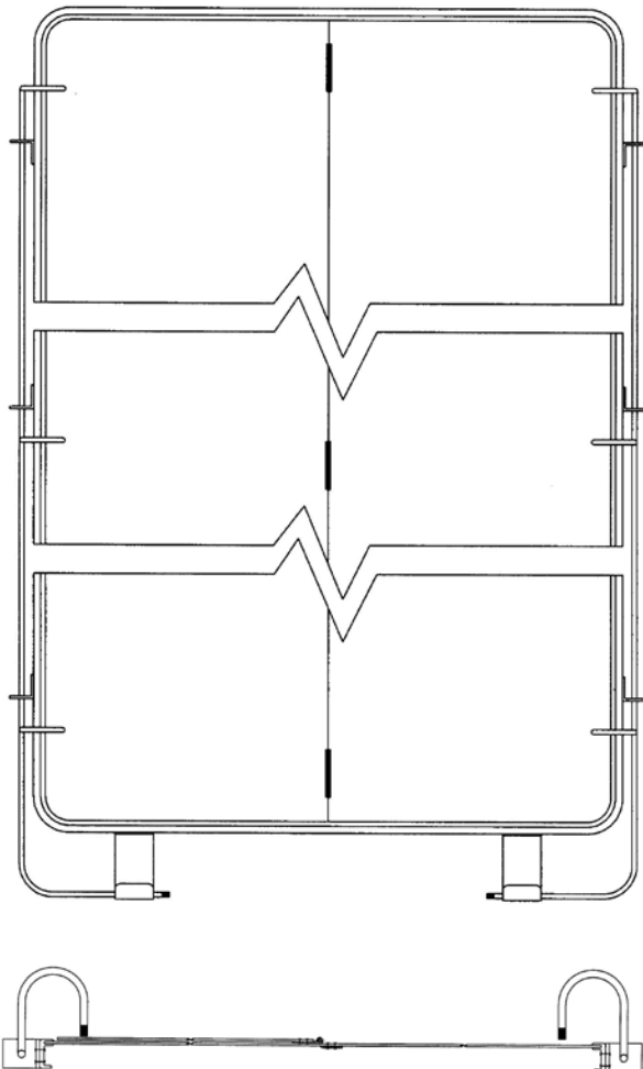
Verriegelungsmechanismus für Buchform mit Edelstahlverriegelung und Grundplatte
